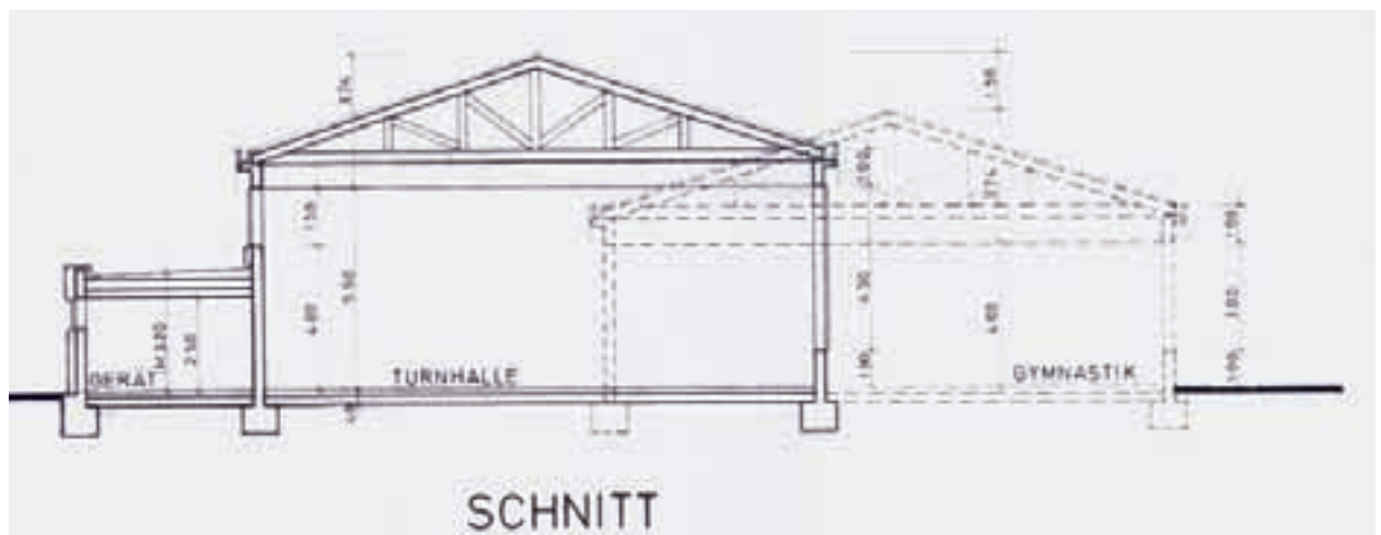
Bild 4.1-7: Schnitt Sporthalle
