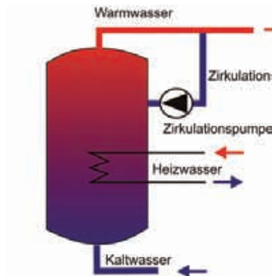
Bild 5.1.9-6: Speicher mit Zirkulationsleitung und -pumpe
