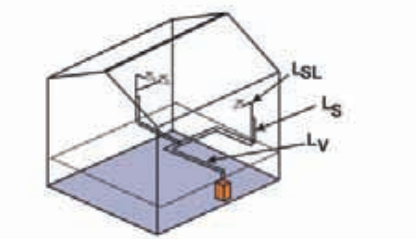
Bild 5.1.9-7: Bezeichnung der Leitungen gemäß DIN V 18599 Teil 8
