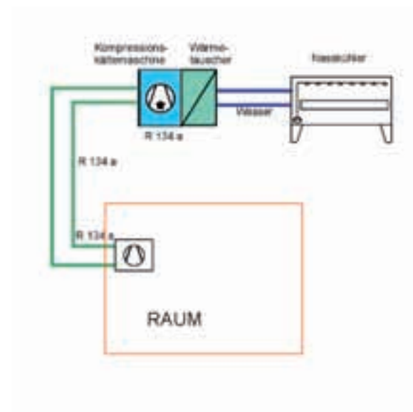
Bild 5.1.8-3: Wassergekühlte Kompressionskältemaschine; Direkte Systeme
