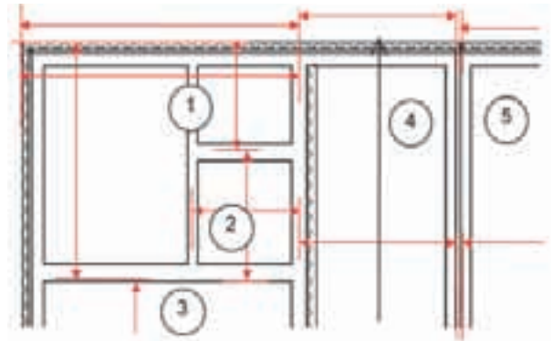
Bild 5.1.2-2: Maßbezüge nach DIN V 18599 Teil 1
